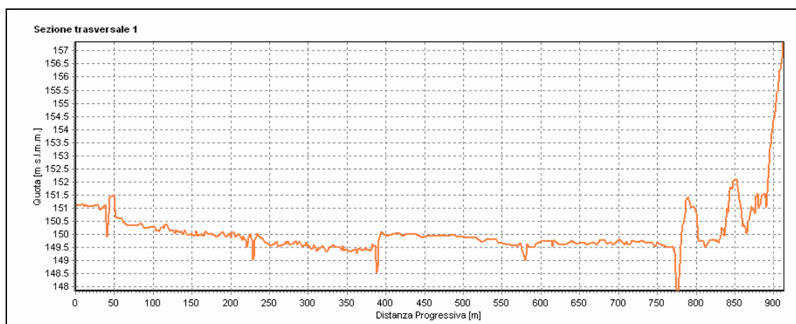
Figura 7.3.2.2: sezione trasversale n. 1 dell'area denominata Paludo
