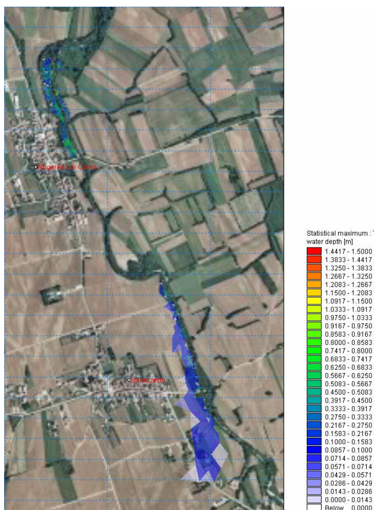
Figura 7.2.2.3: modello numerico di propagazione dell'onda di piena da San Mauro a Codroipo; esondazione nei Comuni di Coseano e Mereto di Tomba, rispettivamente nelle frazioni di Nogaredo di Corno e Barazzetto
