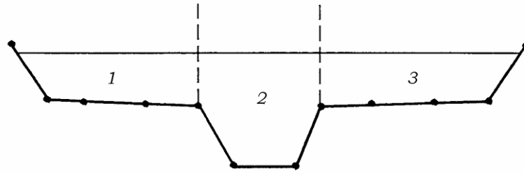
Figura 6.1.2: sezione schematica di un corso d'acqua naturale
