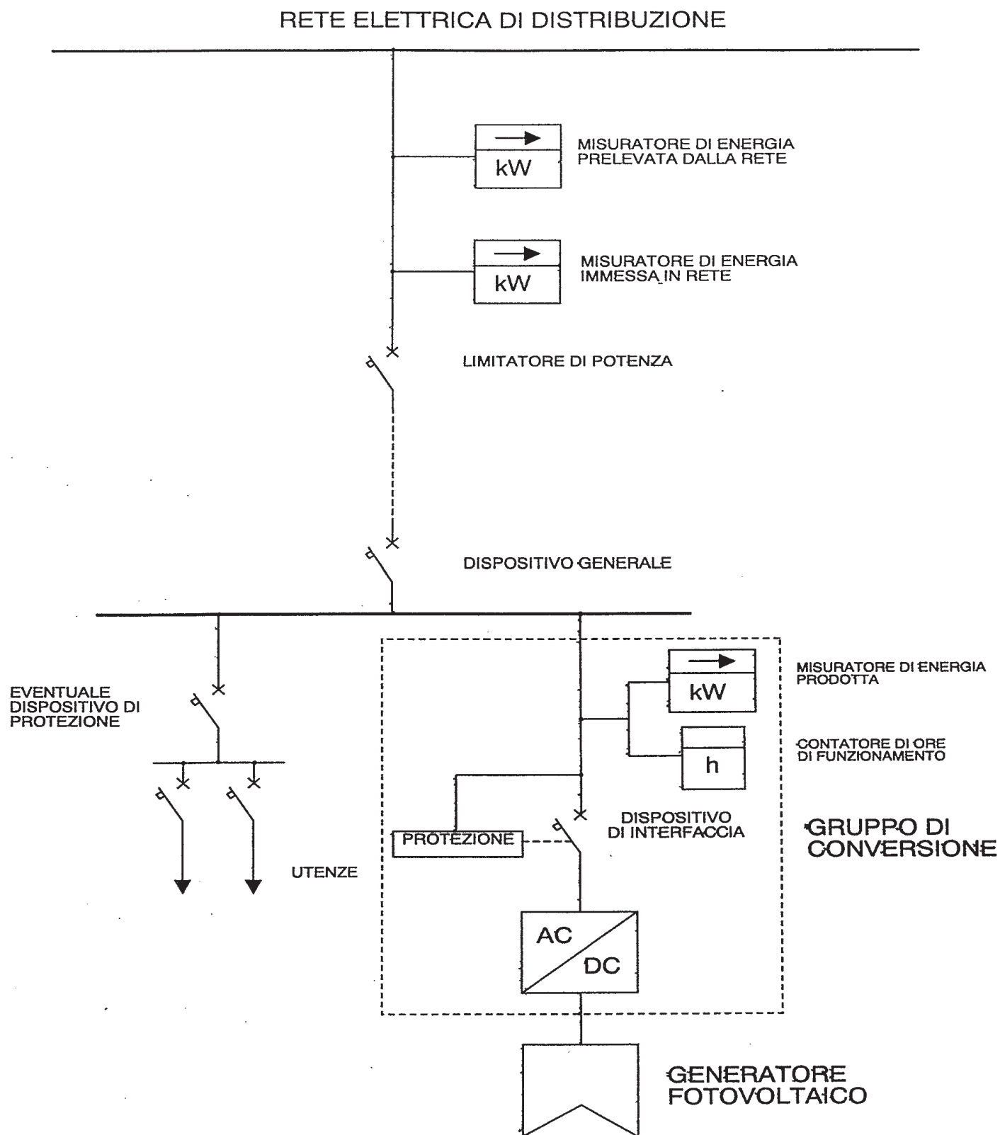
Figura 1: schema tipico di collegamento dell'impianto fotovoltaico alla rete elettrica di distribuzione
